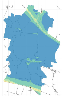
Conc. media annua - Settore: Altro
