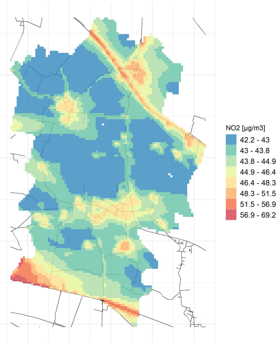
Massima concentrazione giornaliera di NO2
