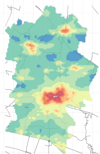
Conc. media annua - Settore: Industria
