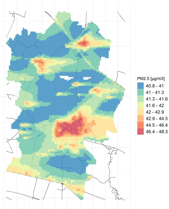
90.4° percentile della conc. media giornaliera di PM2.5
