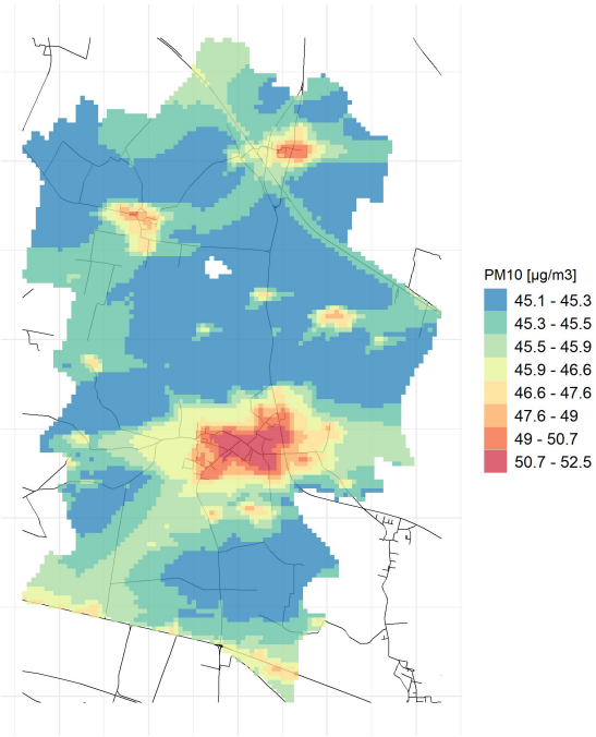
90.4° percentile della conc. media giornaliera di PM10
