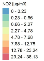
Conc. media annua - Settore: Altro
