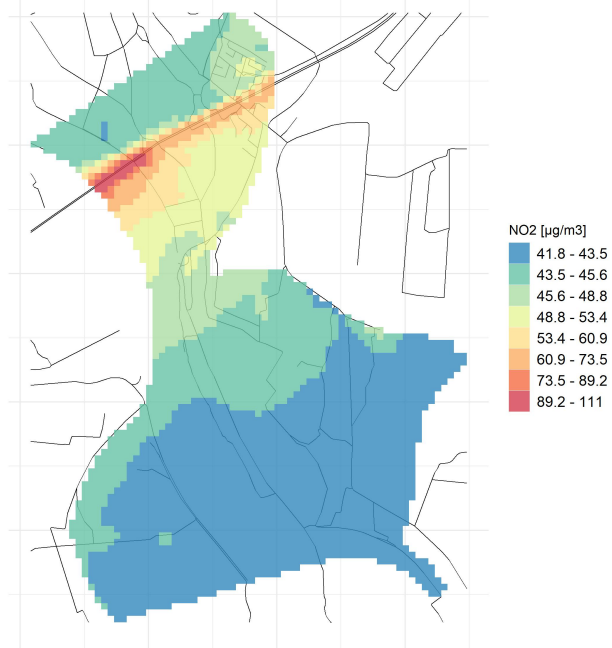
Massima concentrazione giornaliera di NO2
