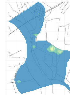
Concentrazione media centro abitato
