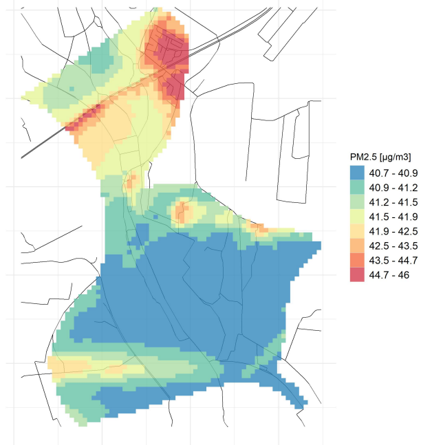
90.4° percentile della conc. media giornaliera di PM2.5
